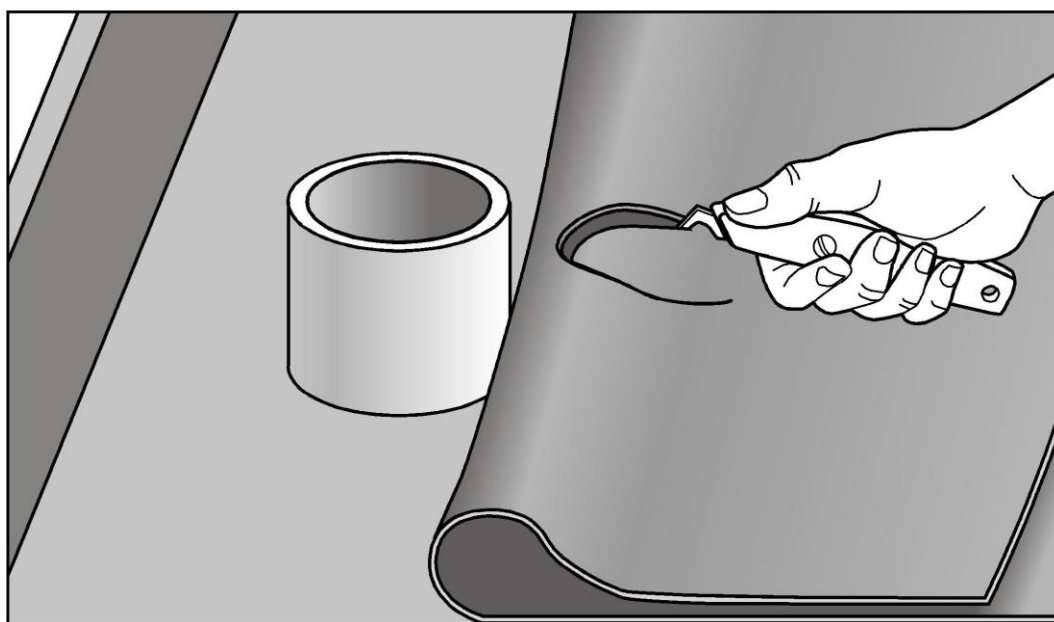
Figur 4. Märk ut och skär hål för krängning.
