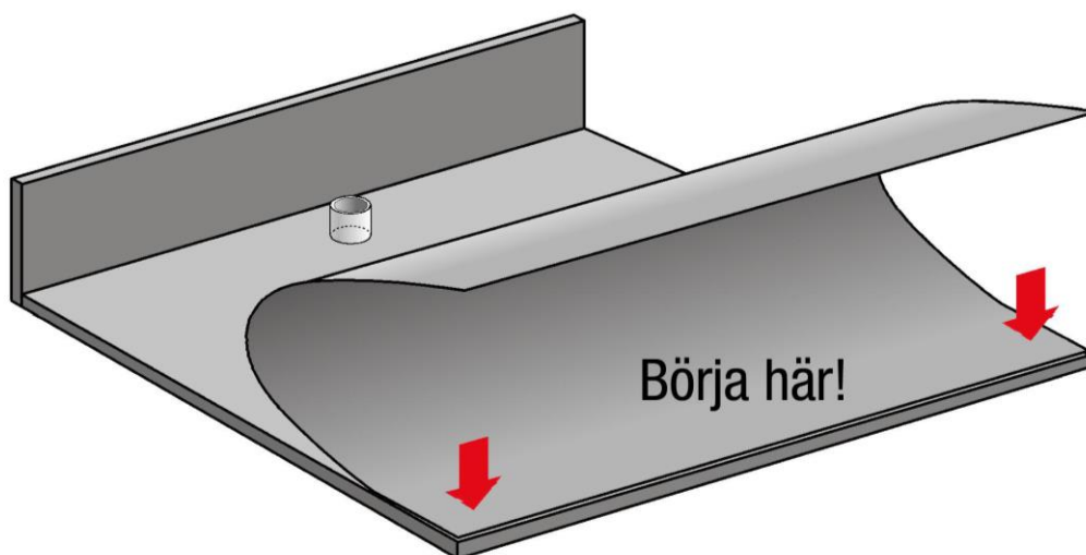
Figur 3. Provbitten ska först fästas i golvet på motsatt sida om väggen.
