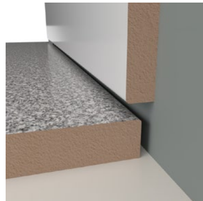
FIGUR 18 B. Golvplatta monterad innan vägglatta.
