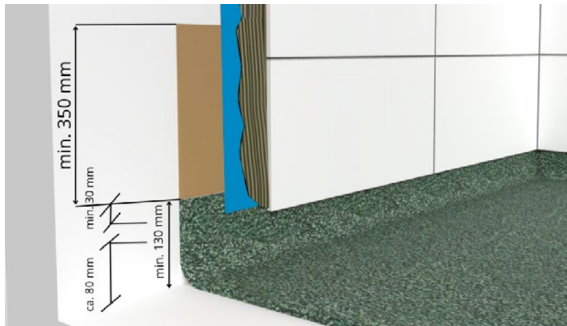
FIGUR 8. Övergång mellan plastmatta på golv och keramik på vägg eller fogfritt golv och keramik på vägg. Vid eventuellt tätskikt ska det vara ett överlapp på minst 30 mm över mattkant.
