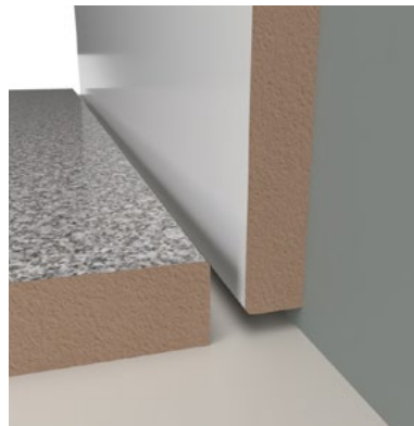
FIGUR 18 A. Vägglatta monterad innan golvplatta.
