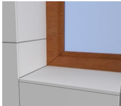
FIGUR 16 B. Smygens platta råder över väggens platta, på sidorna är det väggens platta som råder över smygens platta.
