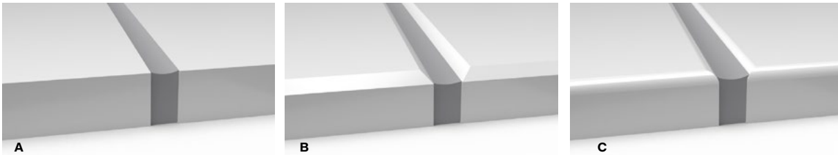
FIGUR 12 A–C. I figurerna ovan visas fogfyllnad för plattor med rak, avfasad respektive rundad kant.
