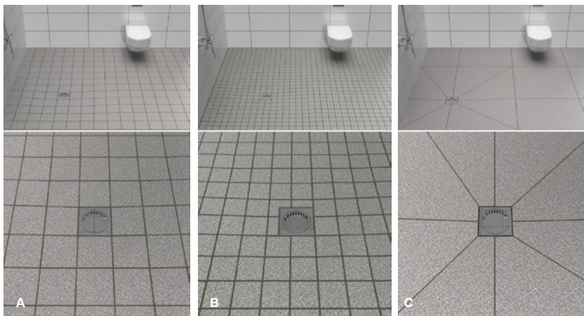
FIGUR 19 A-C. Till höger visas tre sätt att lägga plattor vid fall i duschplats med vanlig brunn.
