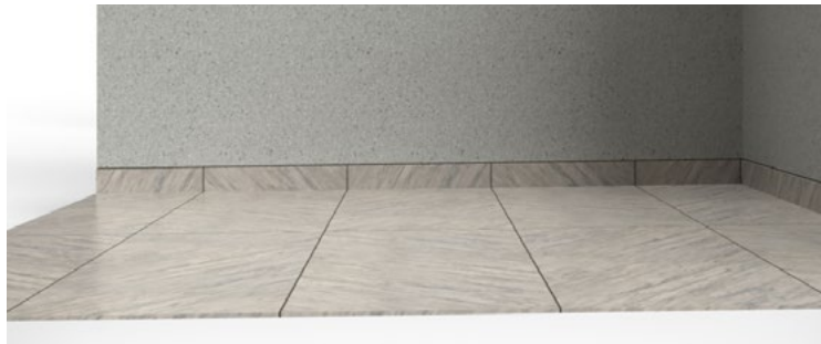
FIGUR 14 B. Sockelplattans övre kant följer golv/väggvinkeln.
