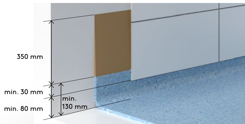
FIGUR 9. Övergång mellan plastmatta på golv och keramik på vägg eller fogfritt golv och keramik på vägg.
