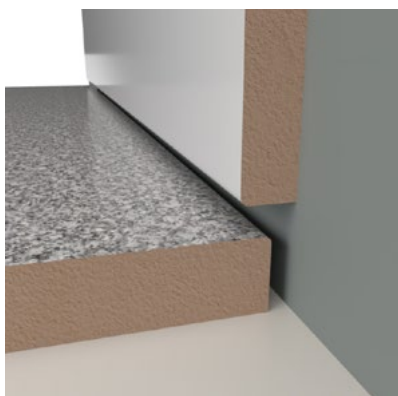
FIGUR 19 B. Golvets platta råder över väggens platta.
