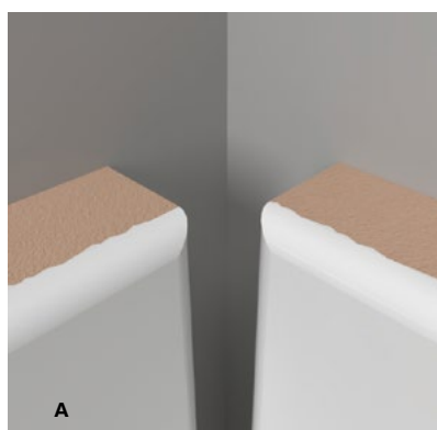
Figur 5 A-B Det finns två alternativ när plattor möts: glasyrkan mot glasyrkan eller att en platta råder över den andra. Platta ska ej sättas stumt mot vägg.
