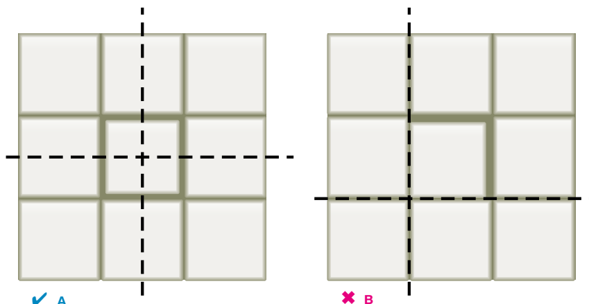
FIGUR 12 A-B. Plattor som är mindre än övriga plattor ska om möjligt centreras.
